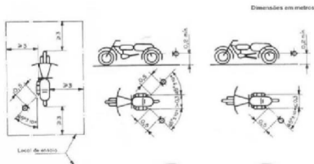
Figura 1: Posicionamento do microfone em relação ao escapamento
